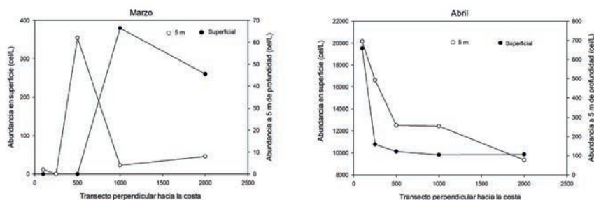
Figura 3 Gráficas de las abundancias de marzo y abril con respecto a la distancia de la costa
