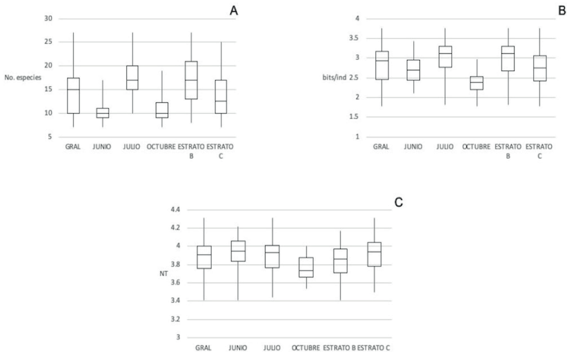
A. riqueza, B. diversidad y C. nivel trófico (C). Mediana (línea horizontal dentro de la caja), valores máximos y mínimos (líneas verticales) y cuartiles.
