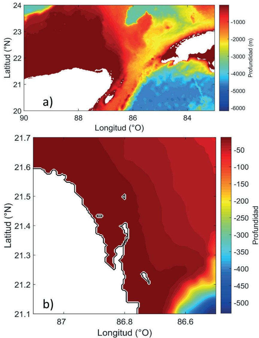
Figura 1 (a) Batimetría del área de estudio regional y (b) batimetría del área de estudio local
